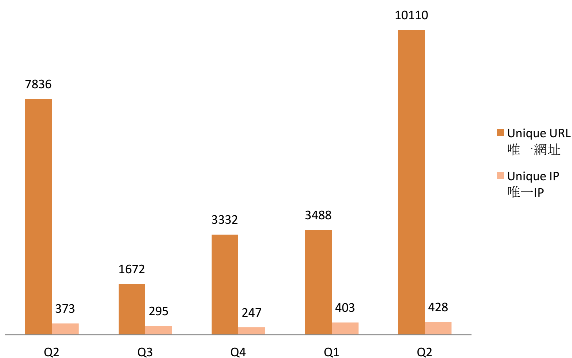
圖 7 - 釣魚網站安全事件趨勢
