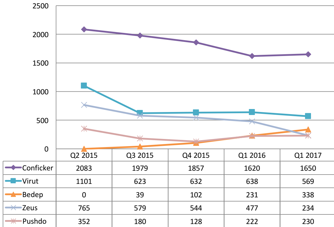
圖 13 -五大主要殭屍網絡趨勢 6
