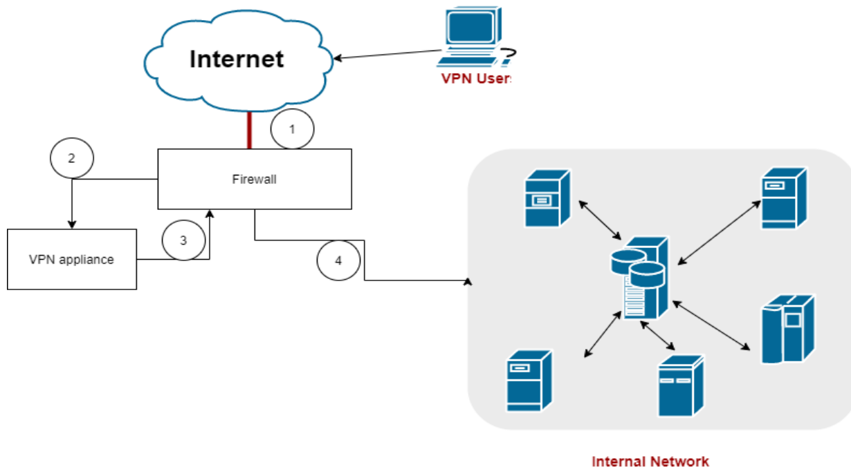
{圖 1 企業 VPN 樣本設計}
